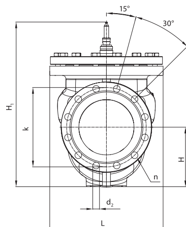
VFM2 DN = 200–250 мм
