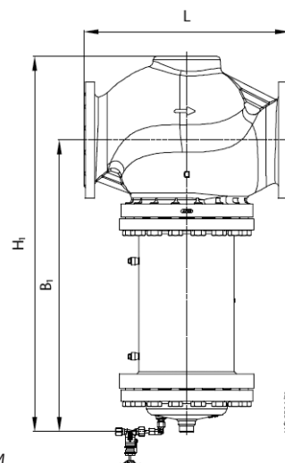
VFG2, VFGS2 DN 150–250 с удлинённым штоком
