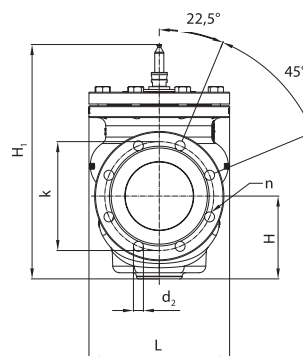
VFM2 DN = 80–150 мм
