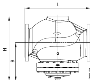
VFG2, VFGS2 DN 150–250 с удлинённым штоком
