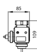
Соединительная деталь K2
