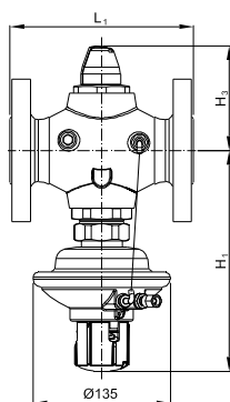
AVPQ DN = 32–50 мм, \Delta P_{\text{рез}} = 0,2\text{--}1,0 бар
