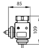
Соединительная деталь K2
