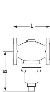
VFG 2 DN = 15–50 мм, VFGS 2 DN = 15–125 мм
