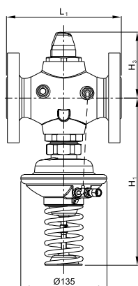
AVPQ DN = 32–50 мм, \Delta P_{\text{рез}} = 0,3\text{--}2,0 бар
