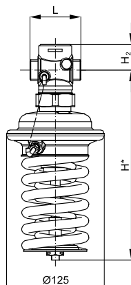
AVD DN = 15–25 мм P рез = 3–12 бар
