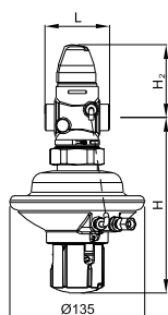
AVPQ DN = 15–50 мм, \Delta P_{\text{рез}} = 0,2\text{--}1,0 бар
