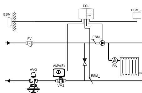
Зависимое присоединение системы отопления к тепловой сети
