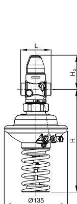
AVPQ DN = 15–50 мм, \Delta P_{\text{рез}} = 0,3\text{--}2,0 бар
