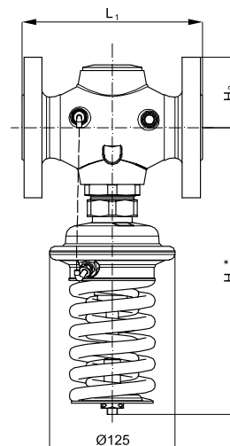
AVD DN = 32–50 мм P рез = 3–12 бар
