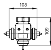
Соединительная деталь K3
