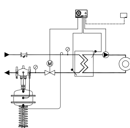
Независимое присоединение системы отопления к тепловым сетям
