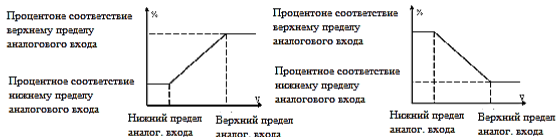
Рис. 6-18 Линейная кривая аналогового входа
