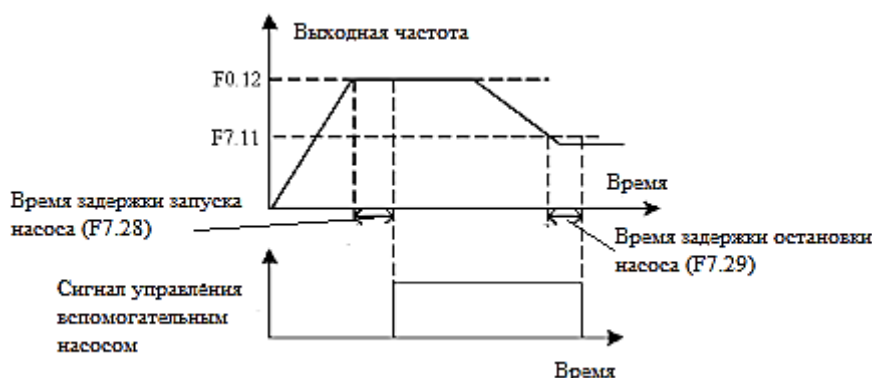
Рис. 6-22 Сигнал управления вспомогательным насосом для постоянной подачи воды под давлением
