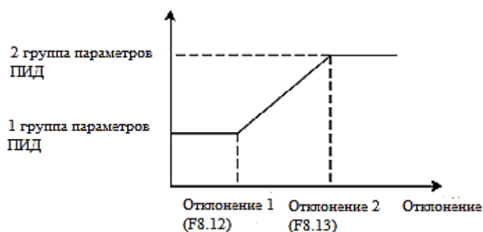
Рис. 6-23 Переключение параметров ПИД
