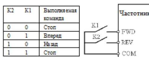
Рис.6-13 Двухпроводной режим управления 1
