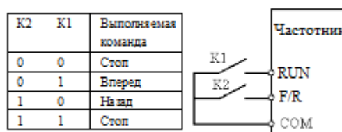
Рис. 6-14 Двухпроводной режим управления 2
