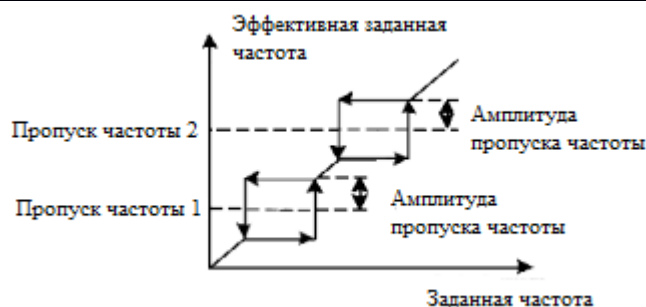
Рис. 6-5 Пропуск частот
