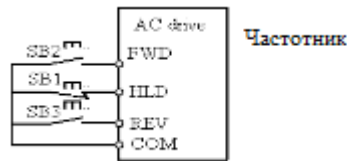
Рис.6-15 Трехпроводной режим управления 1
