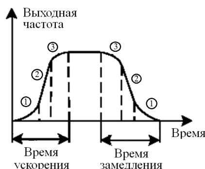
Рис. 6-4 Ускорения/замедление на S-кривой
