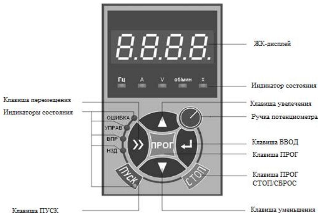
Рис. 4-1 Рисунок панели управления
