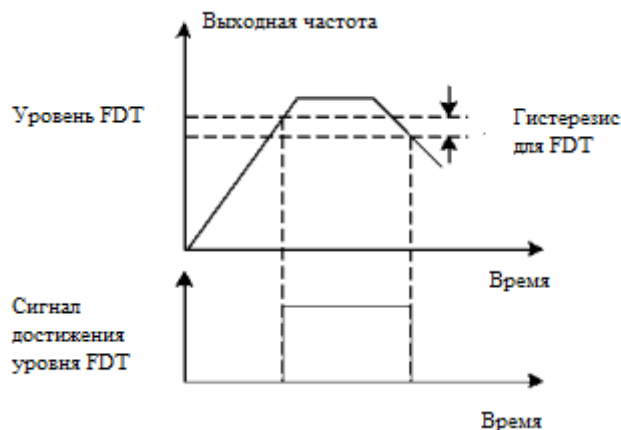
Рис. 6-21 Уровень FDT и схема задержки
