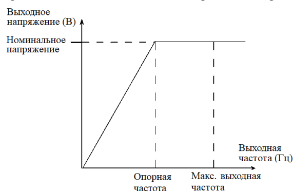
Рис. 6-1 Типичная схема отношения напряжения и частоты
