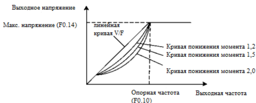
Рис. 6-8 Кривая понижения крутящего момента
