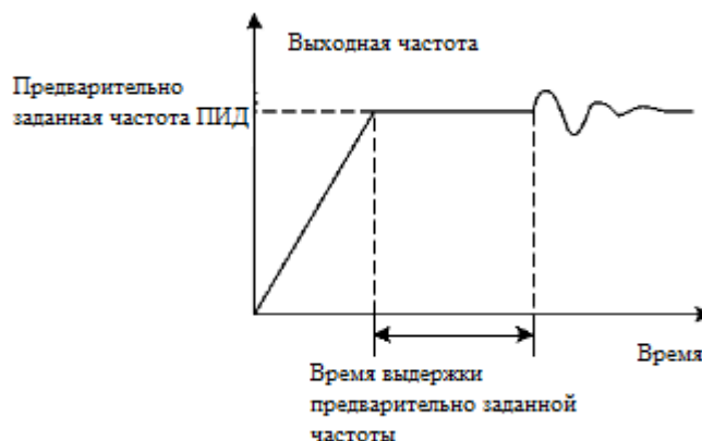
Рис. 6-24 Предварительно заданная частота и время выдержки предварительно заданной частоты ПИД
