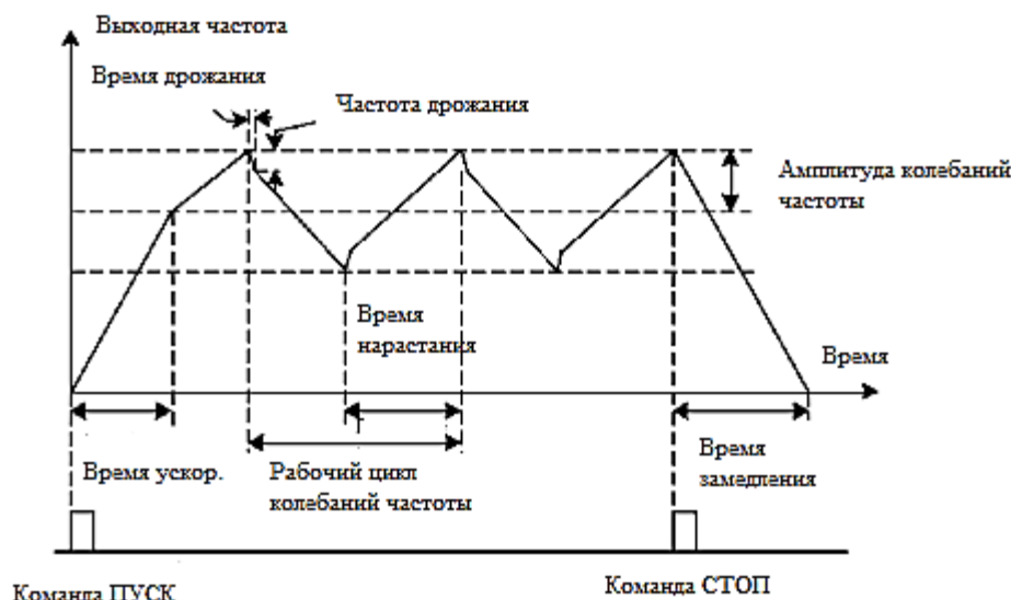
Рис. 6-26 Схема изображения колебаний частоты
