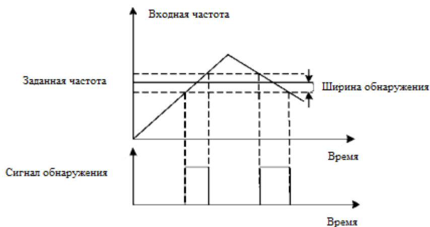
Рис.6-20 Схема обнаружения FAR
