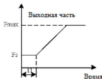
Рис.6-3 Пусковая частота и время выдержки пусковой частоты
