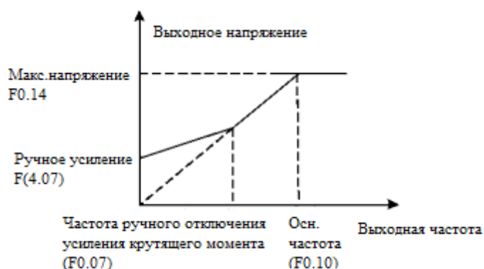
Рис.6-10 Схема усиления крутящего момента
