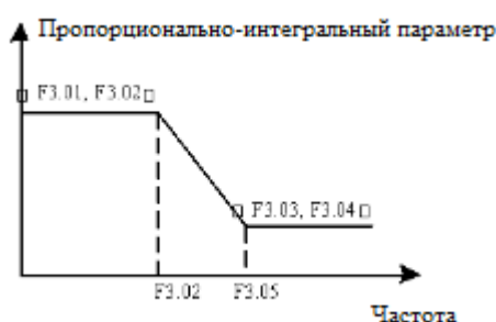
Рис. 6-7 Схема пропорционально-интегральных параметров контура скорости
