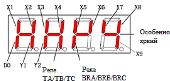
Рис. 6-28 Схема отображения текущего состояния статуса клемм
