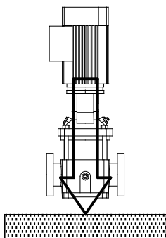
Рис. 2 Правильный монтаж
