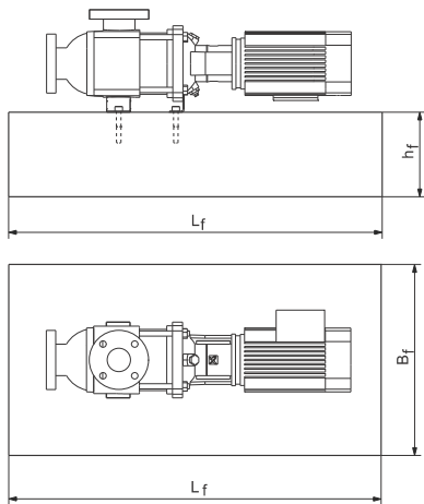
Рис. 4 Фундамент, горизонтальная установка
