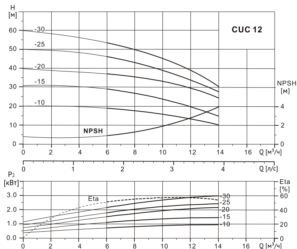
Диаграмма характеристик
