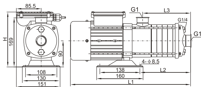
Габаритный чертеж
