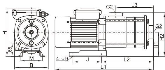
Габаритный чертеж
