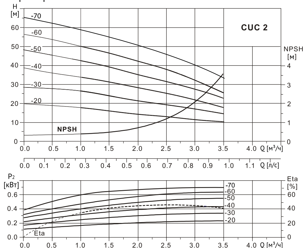
Диаграмма характеристик
