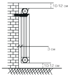
Рис. 2. Правила установки радиатора
