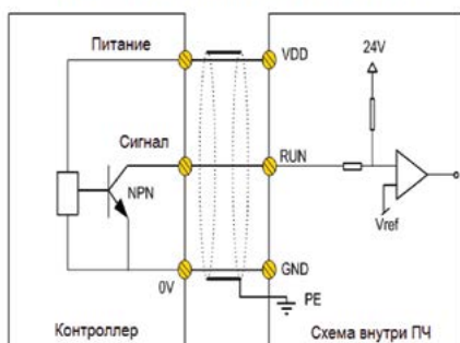
Подключение дискретных входов DI в режиме NPN
