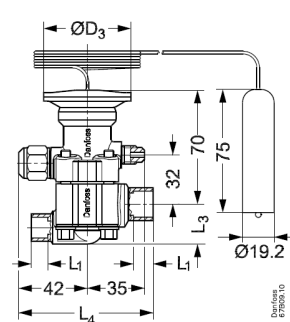
Прямоточный под пайку Вес в сборе ~ 1,0 кг
