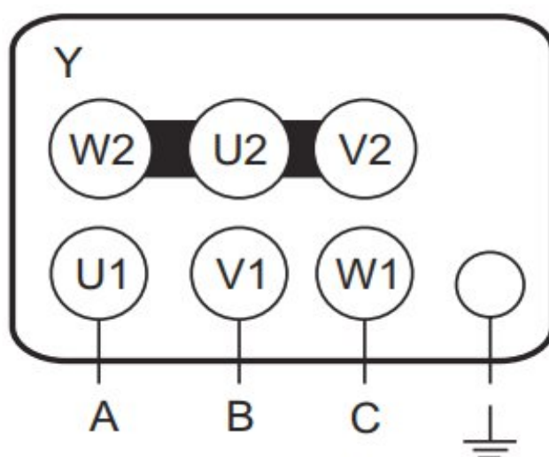
Рисунок А Электрическая схема подключения вентиляторов для сети 380В с номинальным напряжением /Y 220/380 В подключение ЗВЕЗДОЙ
