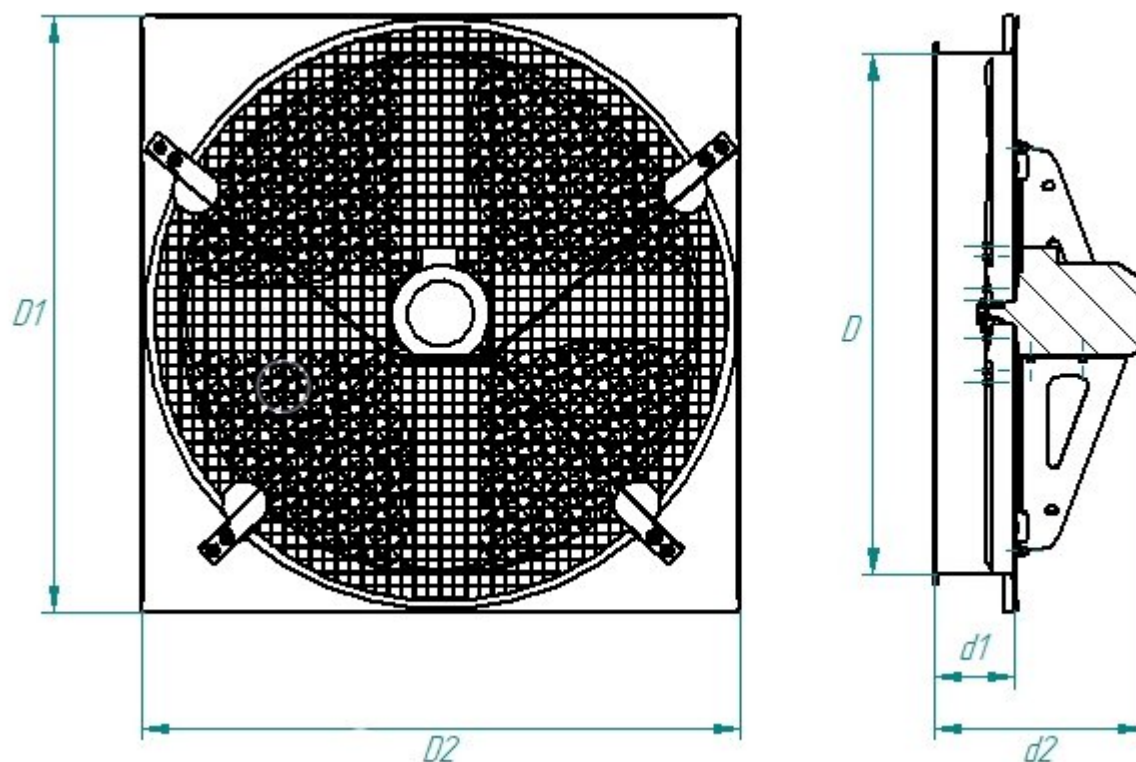
Рисунок 2 Габаритные и присоединительные размеры вентиляторов РВО (D)
