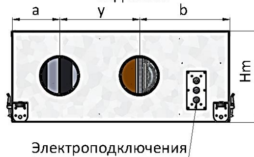
Вид слева
