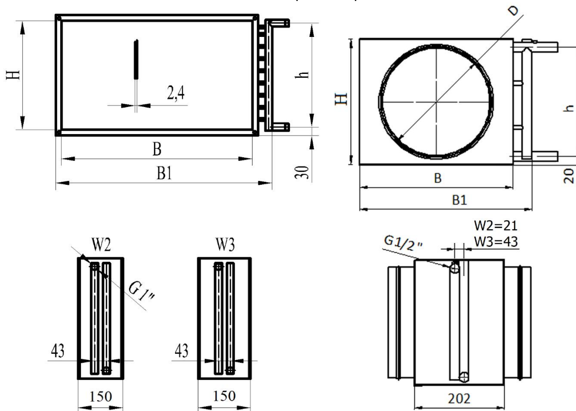
Габариты нагревателей
