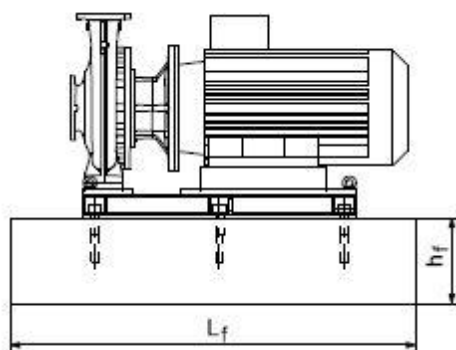
Рис. 4. Фундамент
