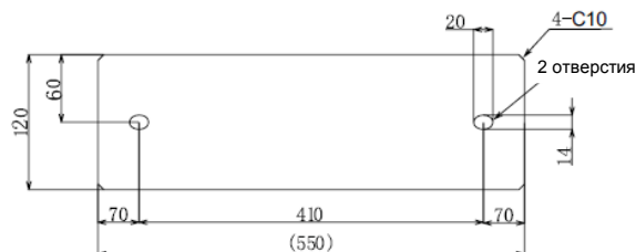
Рис. 4.6 Монтаж рамы и основания
