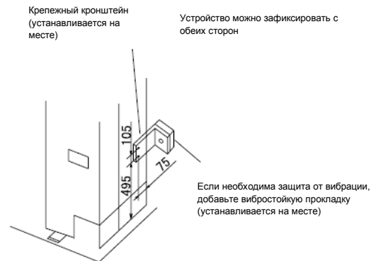
Рис. 4.5 Дополнительное устройство для фиксации
