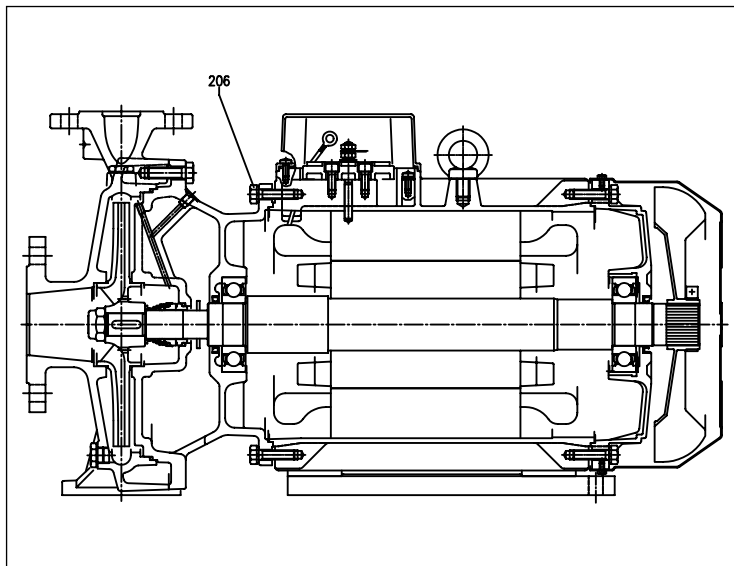
РАЗРЕЗ MD от 15 кВт и более
