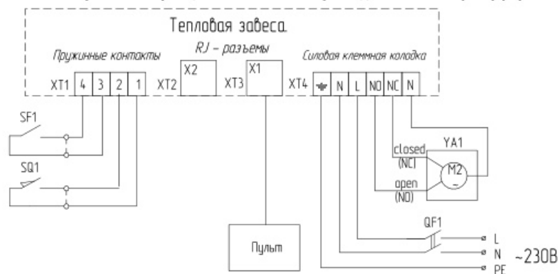
Схема электрическая принципиальная завеса при подключении к пульту управления Ballu BRC-D
