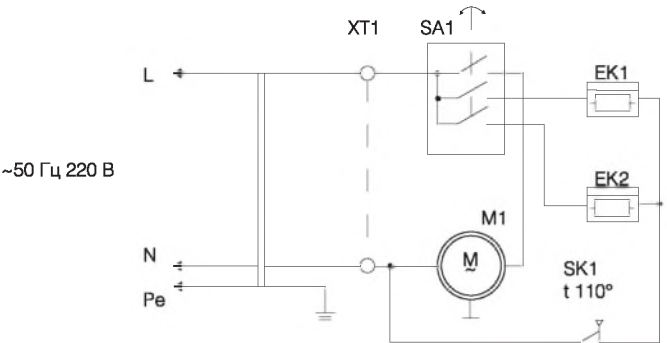
Схема комутации переключателя
