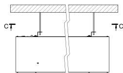
C-C
