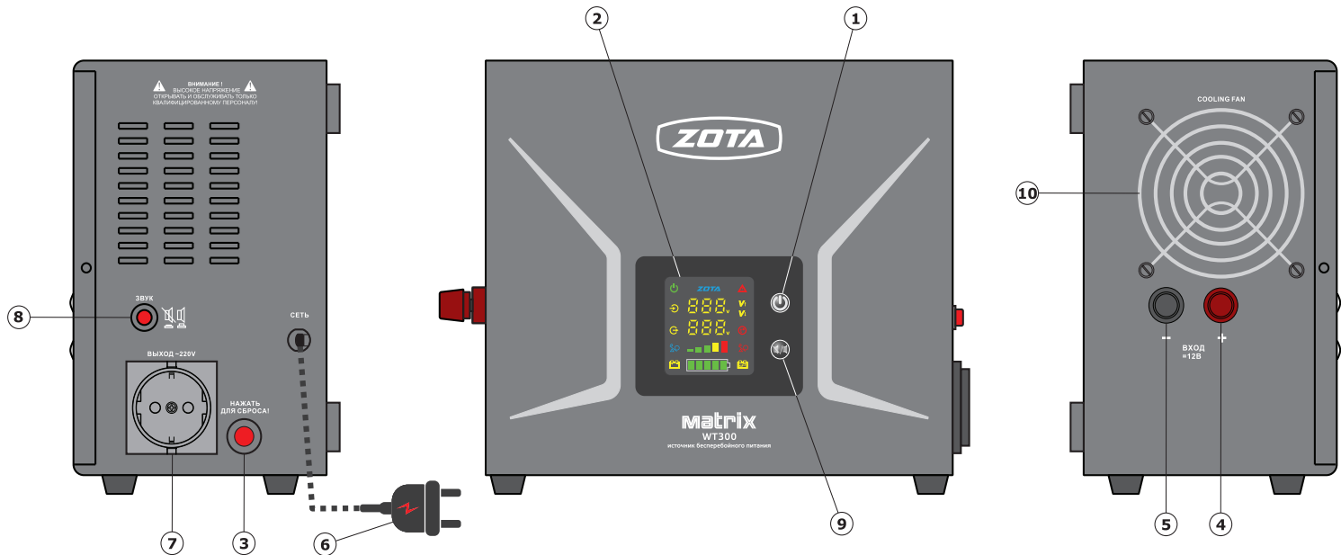
Рис.1 Элементы управления инвертора Matrix-WT300....Matrix-WT1800.
