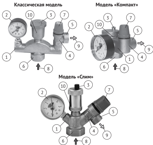
Рисунок 2 - Устройство ГБК
