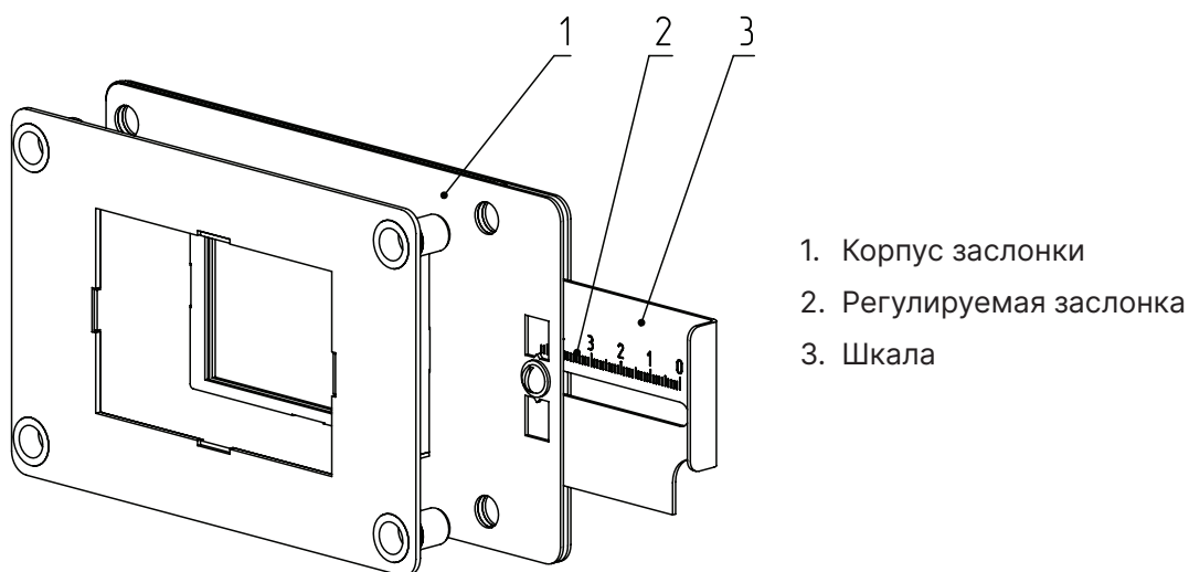
Рис.11 Заслонка вентилятора
