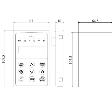
Рис.2-7 Монтажные размеры пульта управления
