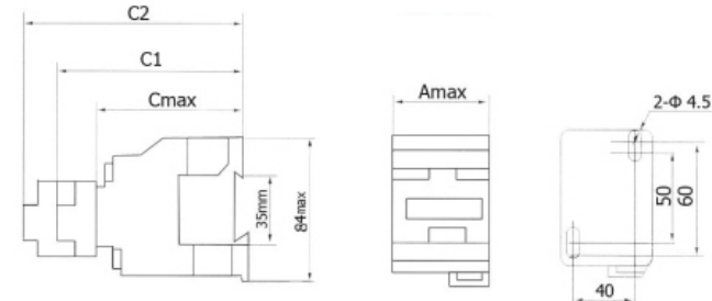
Рисунок 1 – Габаритные и присоединительные размеры пускателей 9 -12А
