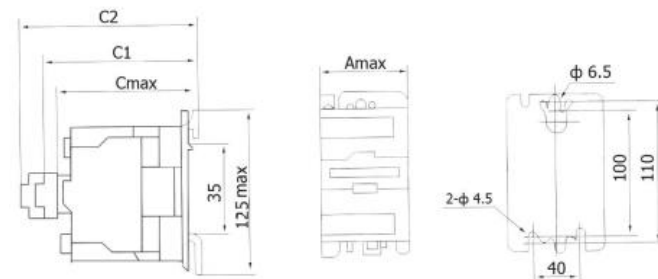
Рисунок 3 - Габаритные и присоединительные размеры пускателей 40 -100А
