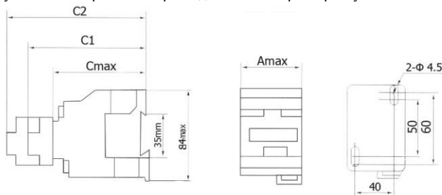
Рисунок 3 - Габаритные и присоединительные размеры пускателей 16-40А
