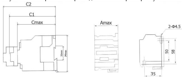
Рисунок 3 - Габаритные и присоединительные размеры пускателей 16-40А
