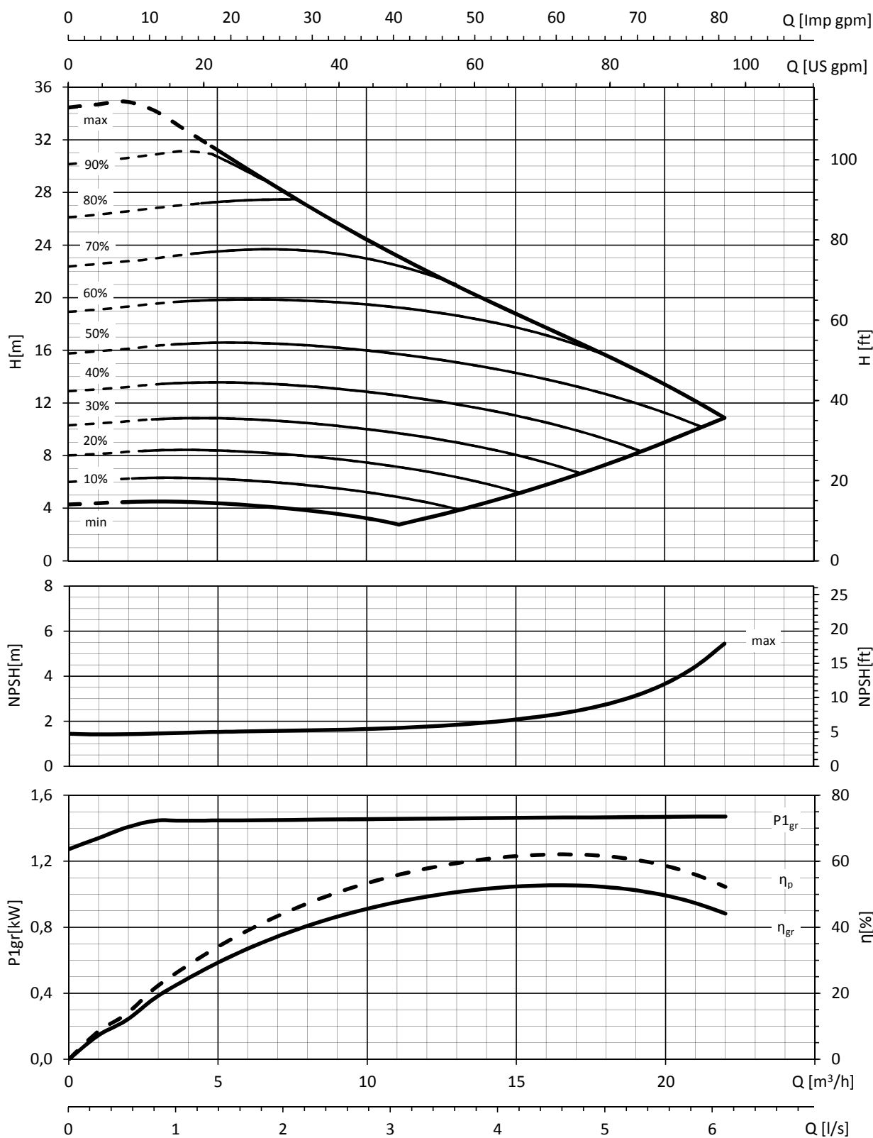
LNE..E 32-160/15/EP02
