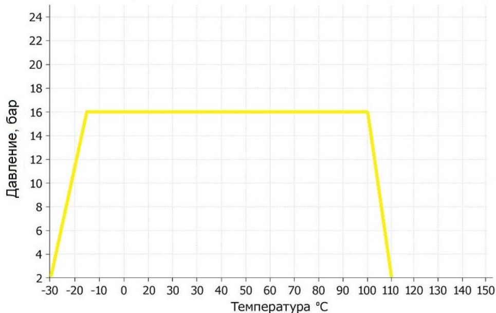
График зависимости температура/давление
