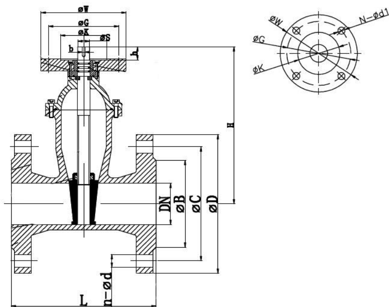
Рисунок 2 - Размеры
