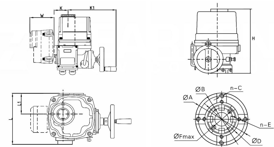
Рисунок 2 - Размеры
