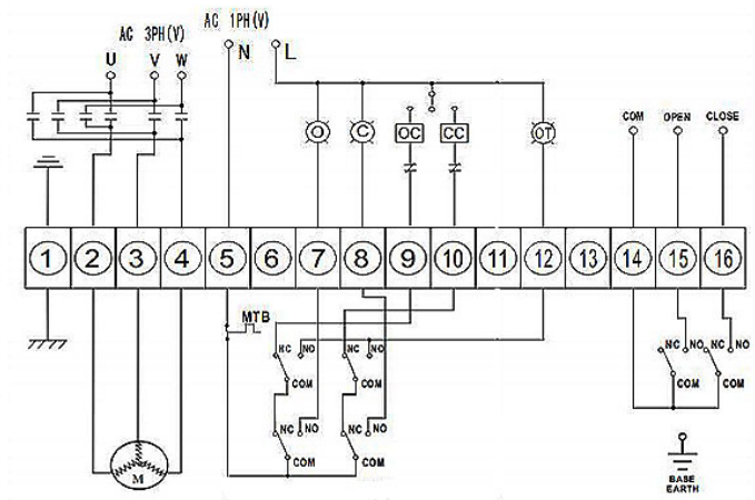
Рисунок 6 - Принципиальная схема подключения электропривода на 380 В
