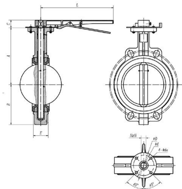
Рисунок 2. Размеры
