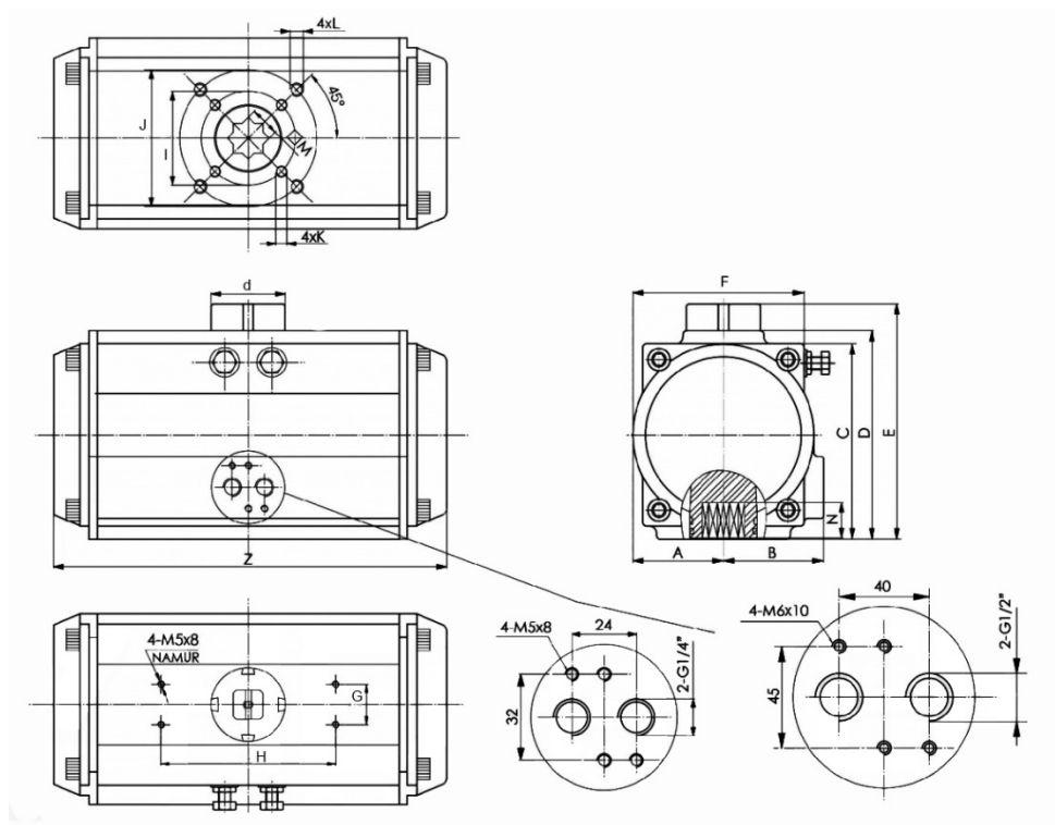
Рисунок 2 – Размеры
