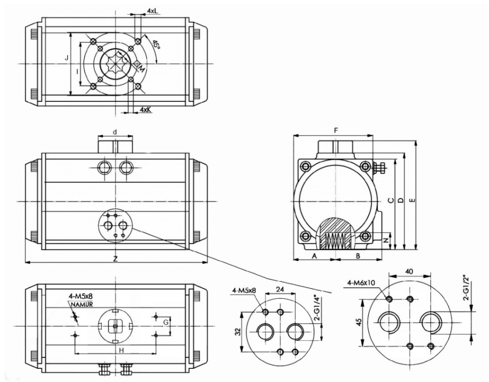
Рисунок 2 – Размеры
