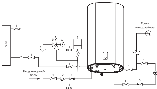
Рис. 4. Вертикальная схема
