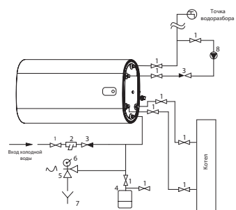
Рис. 5. Горизонтальная схема
