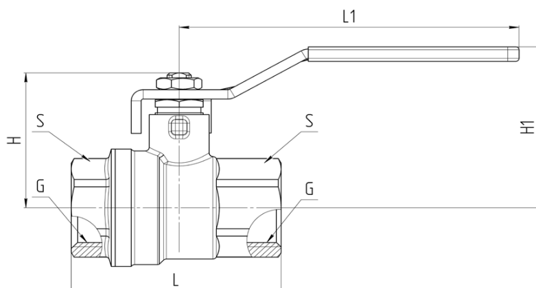
Рисунок 2 – Габаритные размеры крана.
