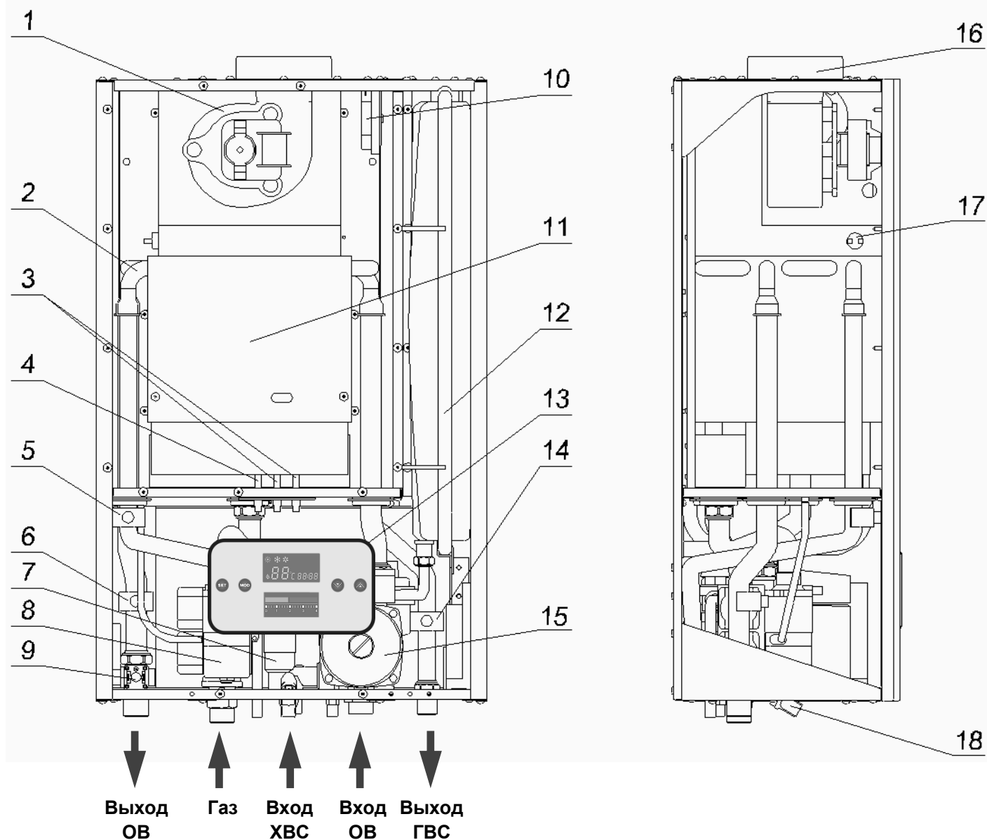
Рис. 4 Устройство котла Amulet (принципиальная схема на примере котла Turbo B)
