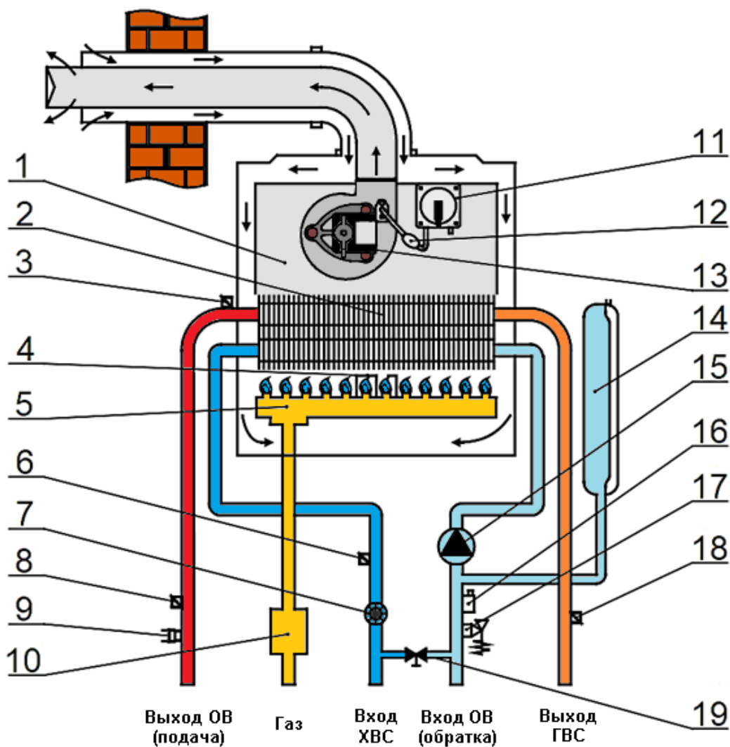
Рис. 1 Функциональная схема котла серии Amulet Turbo B
