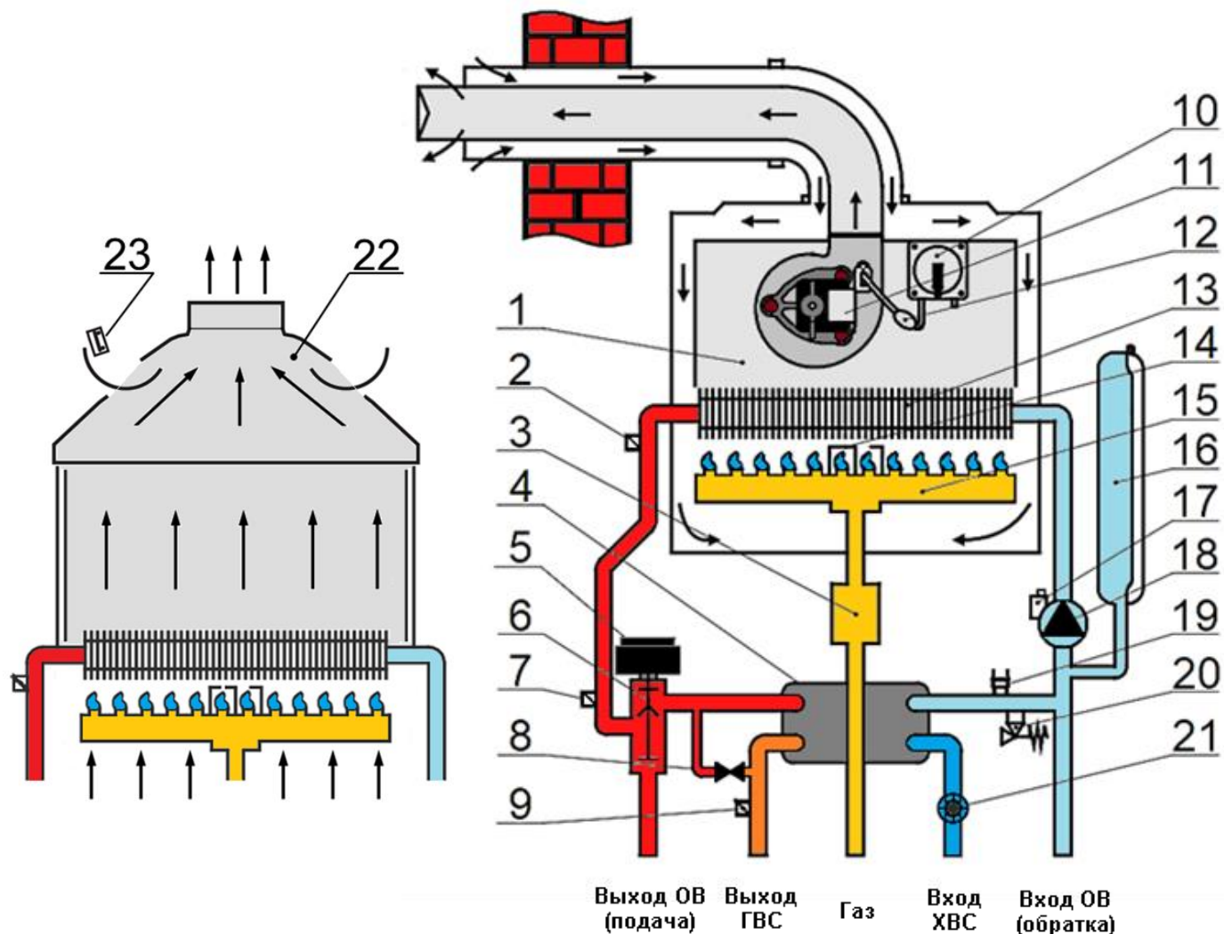
Рис. 2 Функциональная схема котлов серии Amulet Turbo и Amulet Atmo (слева)
