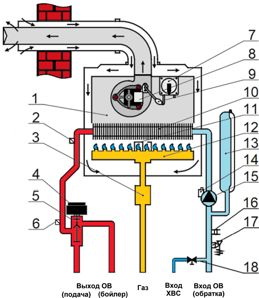
Рис. 3 Функциональная схема котла серии Amulet Turbo SB
