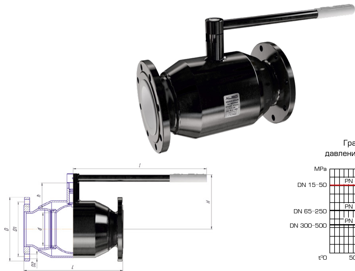
Габаритные и присоединительные размеры:
