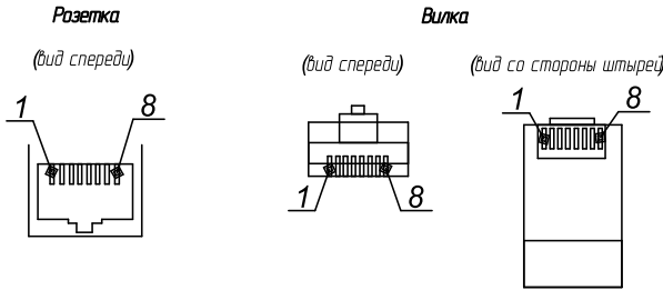
Схема обжимки проводов
