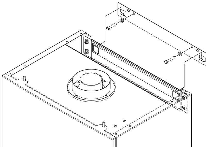
Рис. 18 Монтаж настенного кронштейна
