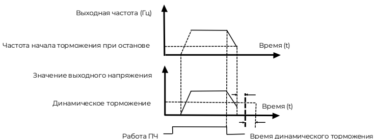
Рисунок 6.5 – Процесс торможения постоянным током
