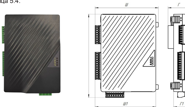
Рисунок 5.7 – Модуль INMX-Ecard
