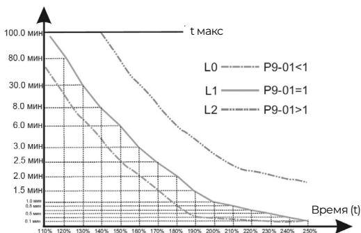
Рисунок 6.18 – Обратнoзависимая времятоковая характеристика
