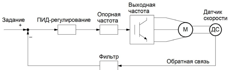
Рисунок 6.20 – Схема ПИД-регулирования
