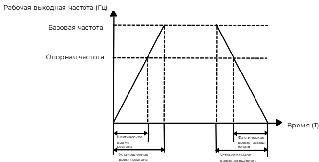
Рисунок 6.3 – Время разгона/замедления
