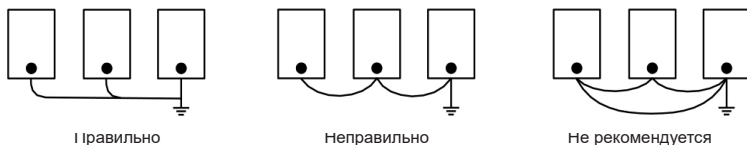
Рис. 3.5 — Схематичное изображение образования петли с заземляющим проводом
