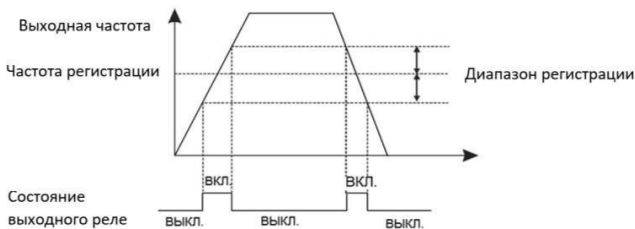
Рис. 6.20 — Зависимость состояния выходного реле от диапазона частоты
