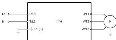
Рис. 3.2.3 — Подключение силовых клемм для моделей LCI-GY/PY-3
