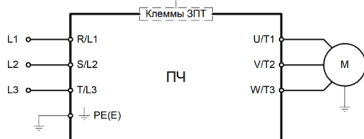
Рис. 3.2.4 — Подключение силовых клемм для моделей LCI-GY/PY-4(B)
