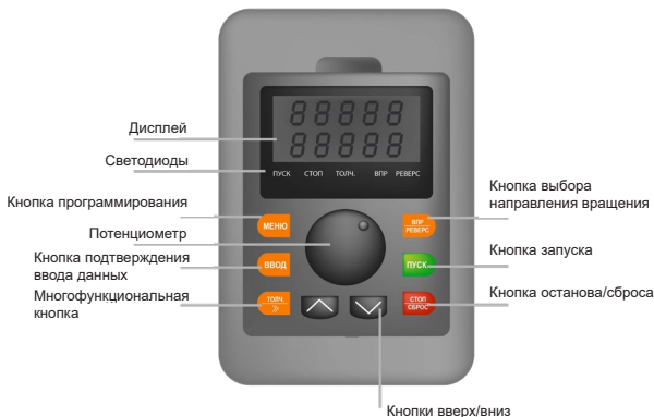
Рис. 5.1 – Функции кнопок и светодиодов панели управления LCI
