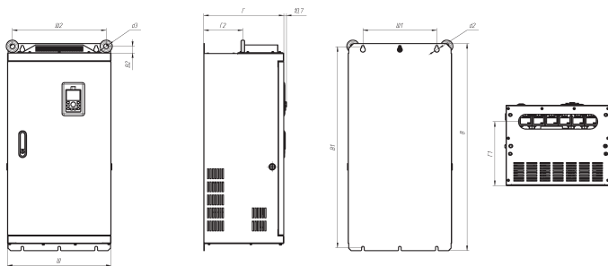
Рис. 2.6 — Габаритные и установочные размеры устройств серии LC1 в металлическом корпусе
