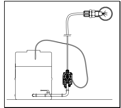
Рис.6: Монтаж на всасывающей трубе
