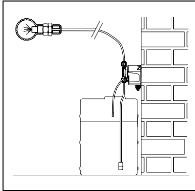
Рис.5 Монтаж на стене
