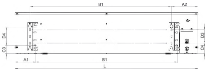
Расположение кронштейнов для вертикальной установки
