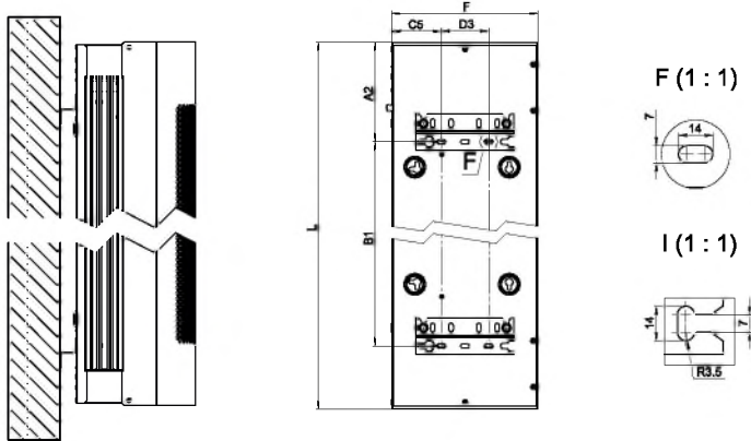
Расположение кронштейнов для вертикальной установки
