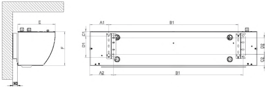
Расположение кронштейнов для установки завесы на шпильки
