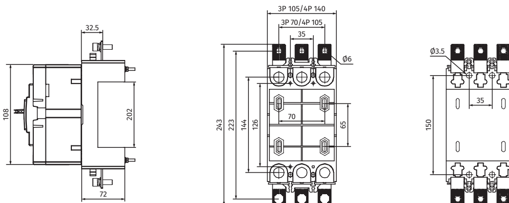
3/4 полюса
