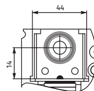
Размеры силового вывода
