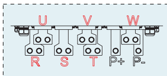
Рисунок 3-26. Схема силовых клемм ПЧ мощностью 280-400 кВт
