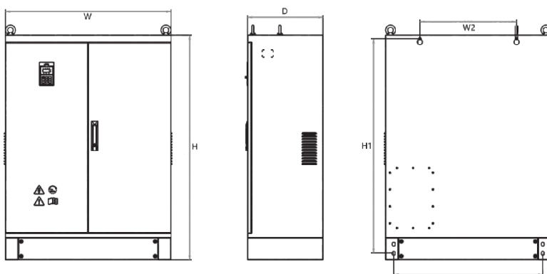
Рисунок 2-12. Габаритные и монтажные размеры ПЧ мощностью 132-400 кВт
