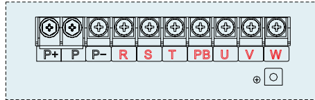
Рисунок 3-10. Схема силовых клемм ПЧ мощностью 22-30 кВт
