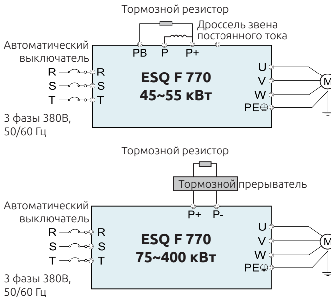
Рисунок 3-18. Основные способы подключения (IP 54).
