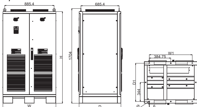
Рисунок 2-10. Габаритные и монтажные размеры ПЧ мощностью 630-710 кВт
