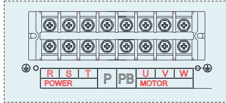
Рисунок 3-11. Схема силовых клемм ПЧ мощностью 37 кВт
