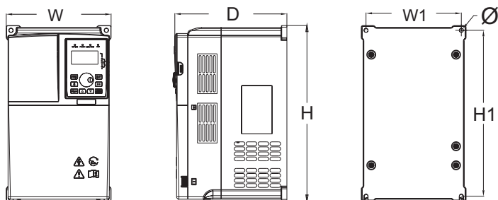
Рисунок 2-13. Габаритные и монтажные размеры ПЧ мощностью 0.75-5.5 кВт
