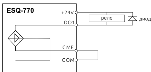
Рисунок 3-29. Схема подключения реле к выходу DO1.
