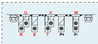
Рисунок 3-24. Схема силовых клемм ПЧ мощностью 132-185 кВт
