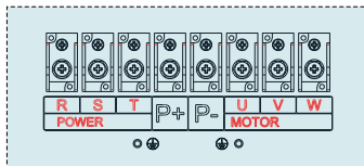
Рисунок 3-23. Схема силовых клемм ПЧ мощностью 70-110 кВт
