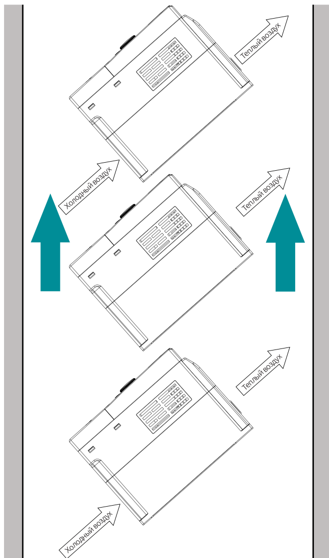
Рисунок 3-6. Диагональная установка.
