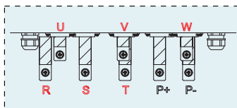
Рисунок 3-25. Схема силовых клемм ПЧ мощностью 200-250 кВт
