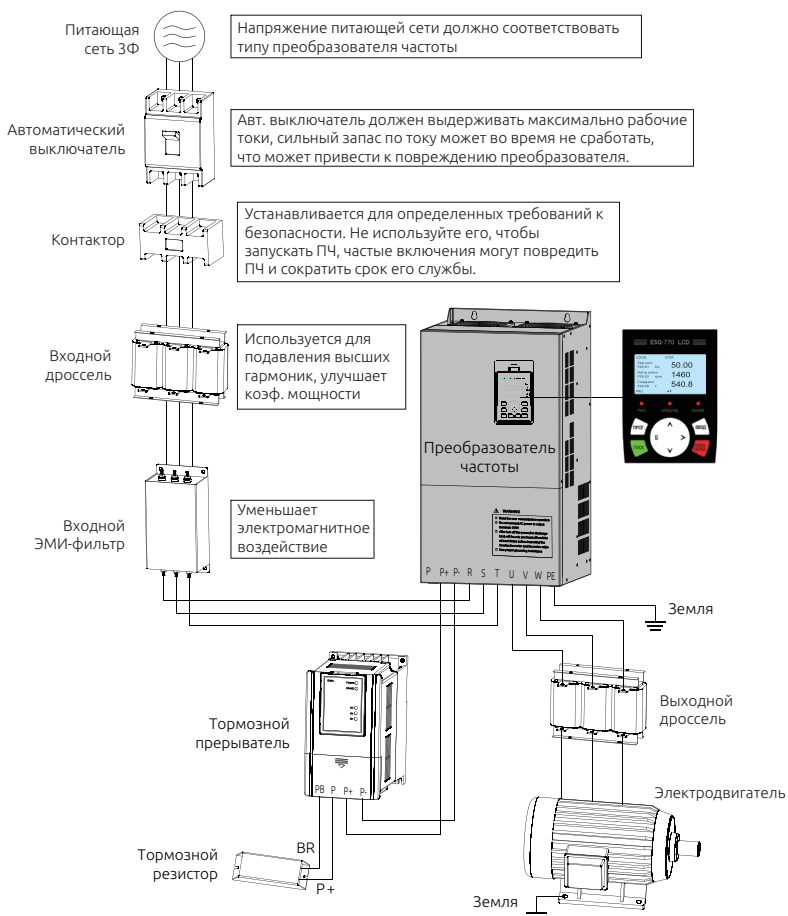
Рисунок 2-13. Структурная схема дополнительного оборудования.
