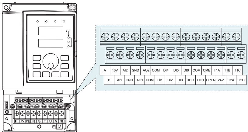
Рисунок 3.24.1 Клеммы управления 0.75-4 кВт
