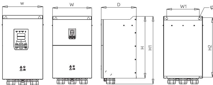
0.7-37 кВт 45-110 кВт
