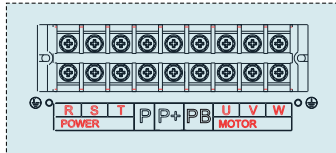
Рисунок 3-22. Схема силовых клемм ПЧ мощностью 45-55 кВт
