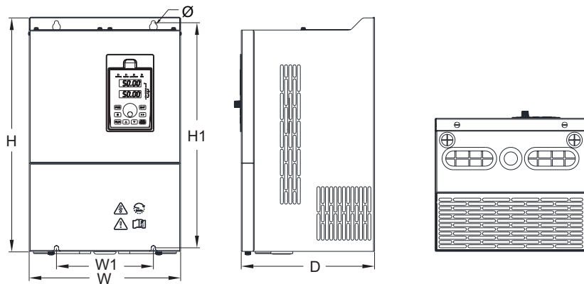
Рисунок 2-14. Габаритные и монтажные размеры ПЧ мощностью 30 – 110 кВт
