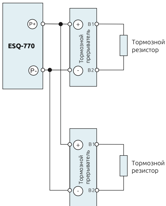
Рисунок 2-16. Параллельное подключение тормозных прерывателей
