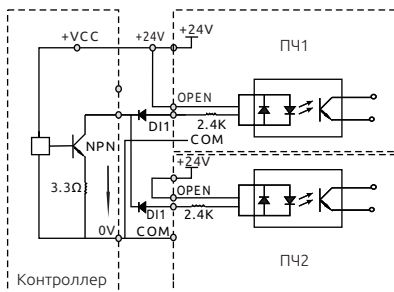
Рисунок 3-27. Параллельное подключение дискретных входов разных ПЧ.
