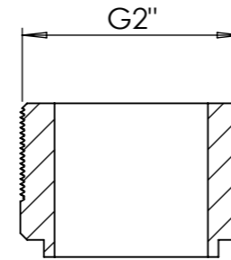
SECTION D-D
