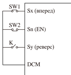
Рисунок 20, 3-проводное управление 2
