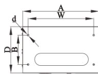
№3. Шкафное исполнение, металл
