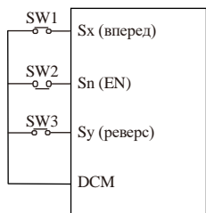
Рисунок 19, 3-проводное управление 1
