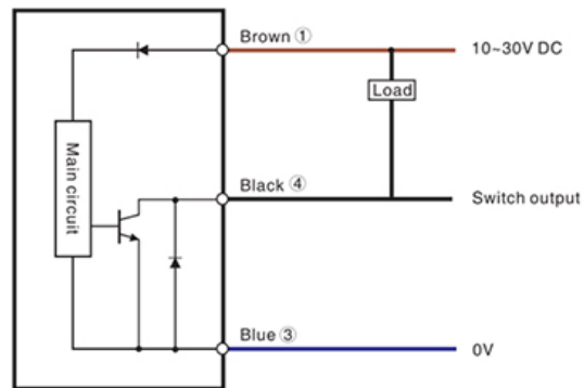
NPN Output
