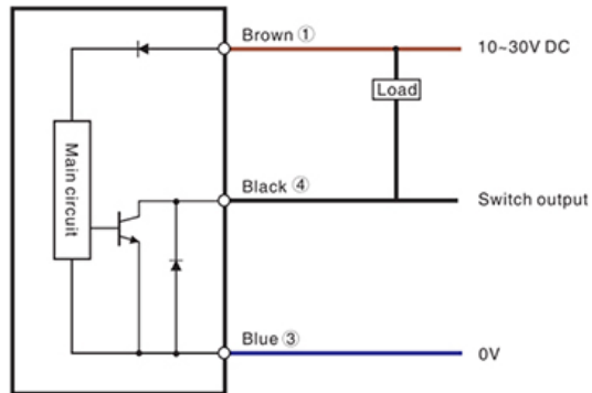
NPN Output
