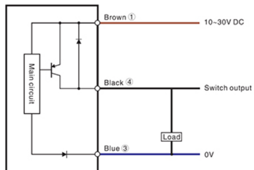
PNP Output
