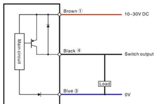
PNP Output
