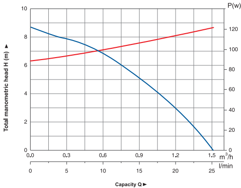
ERP15-90A/160 — Q-H — Q-P
